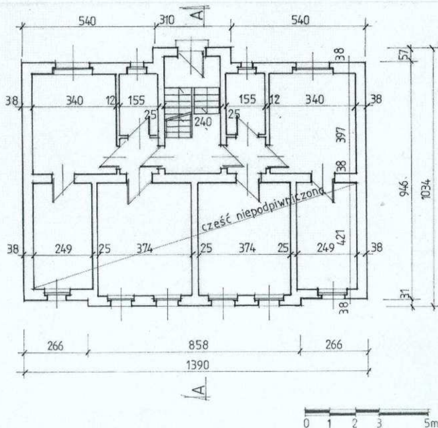
Ryc.4. Rzut parteru.
